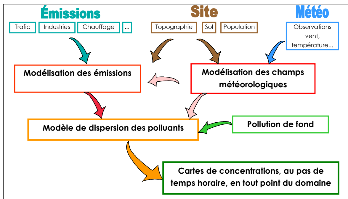
Figure 2 : Principe général de la chaîne de modélisation
