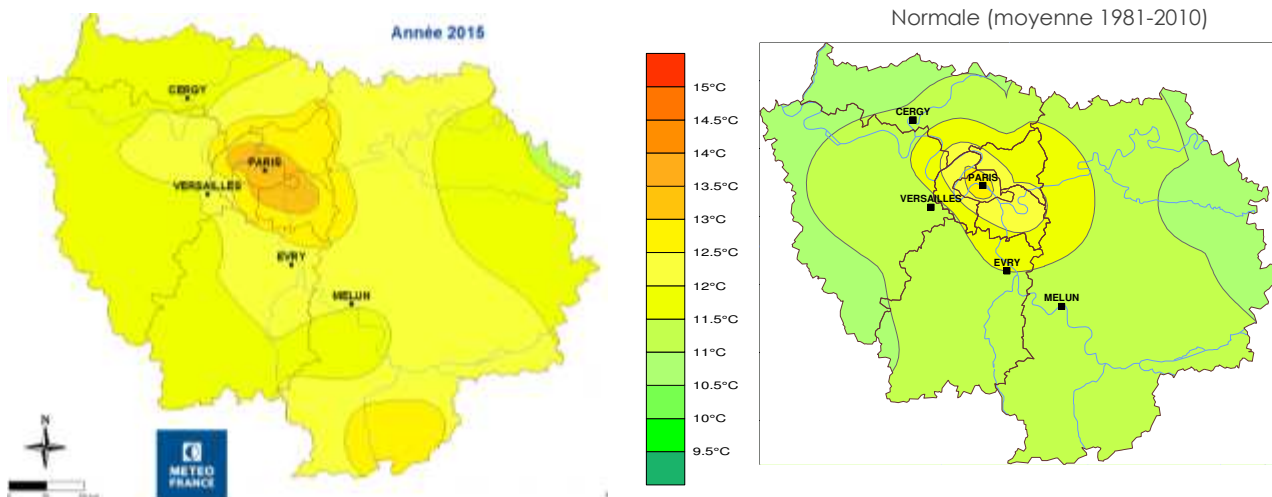
Figure 3 : température moyenne annuelle en Île-de-France (source Météo-France/DIRIC)
